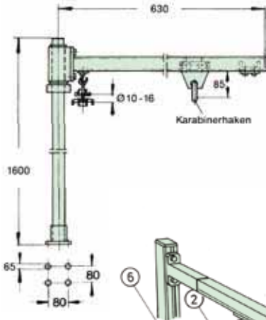
Sekil 1 Döner kollu tripod
