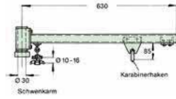
Sekil 2 Ek döner kol
